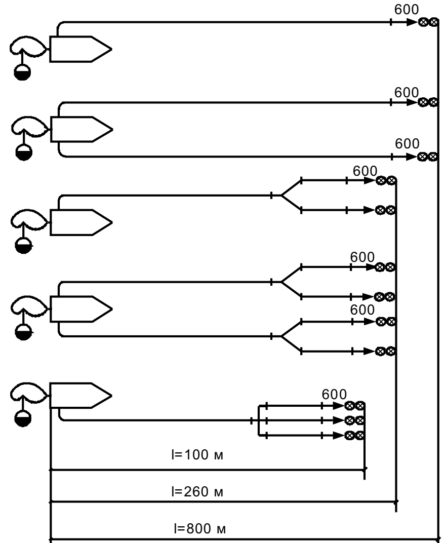
Рис. 4.2. Схемы боевого развертывания АЦ и АН при подаче пены
