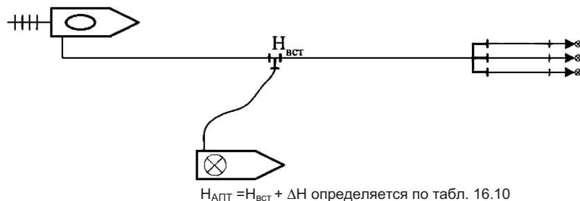
Рис. 16.9. Подача пенообразователя от АПТ в магистральную линию (МЛ), подающую воду от насоса пожарного автомобиля, установленного на водоисточник
