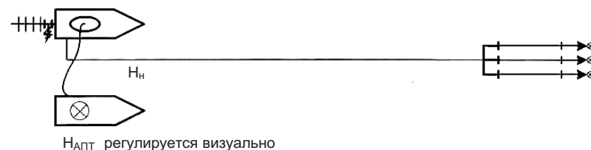
Рис. 16.8. Подача пенообразователя от АПТ в емкость для пенообразователя пожарного автомобиля, подающего пенные стволы
